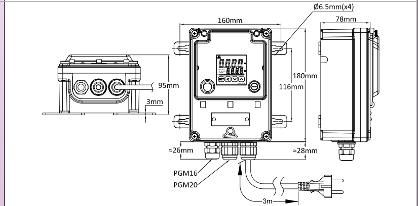
Modèle à 3 presse-étoupes
