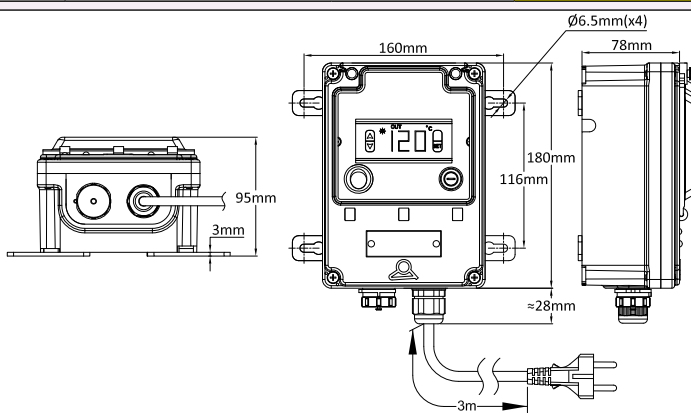
Modèle avec connecteur à 5 voies
