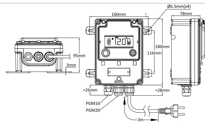
Modèle à 3 presse-étoupes
